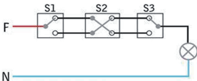
Figura 1: Diagrama do circuito (Fonte: http://equipedeobra.pini.com.br )
